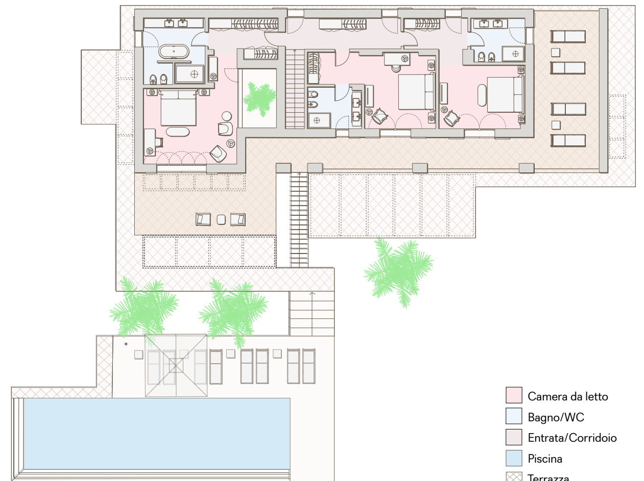
PRIMO PIANO
